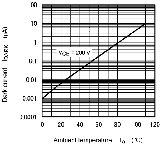
Fig. 11.9 I_{DARK} - T_a
